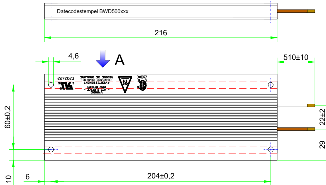
Ansicht A
